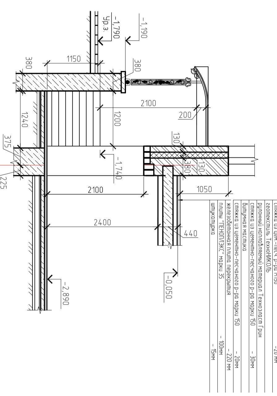
Сечение 1-1
